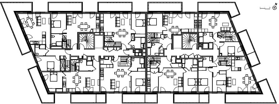
Plan R+9 (duplex niveau bas)
