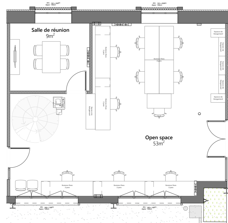
Plan de l'espace proposé
